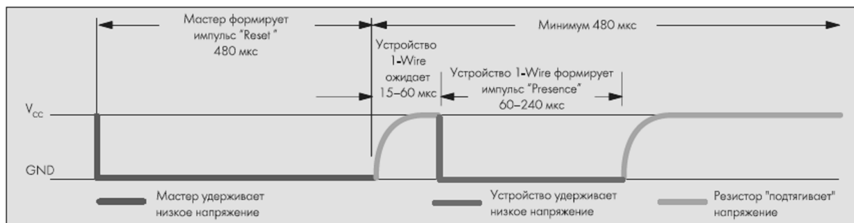
Рис. 2. Последовательность инициализации шины 1-Wire
