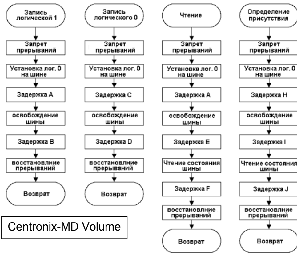
Рис. 3. Функции передачи бит
