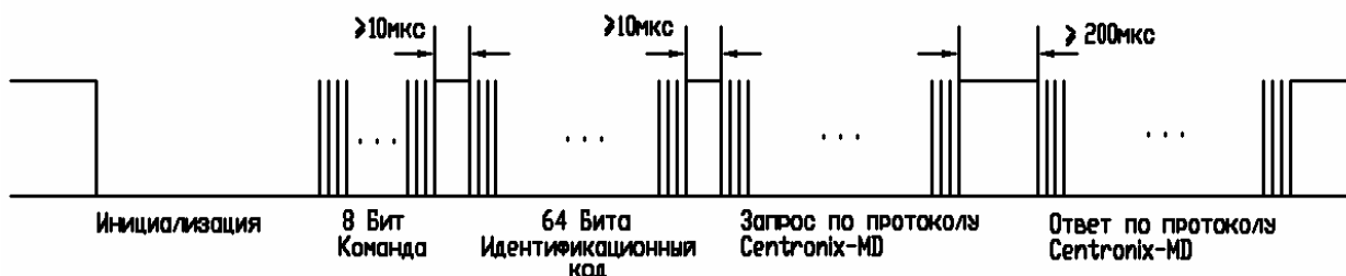
Рис.1. Обмен по шине 1-Wire
