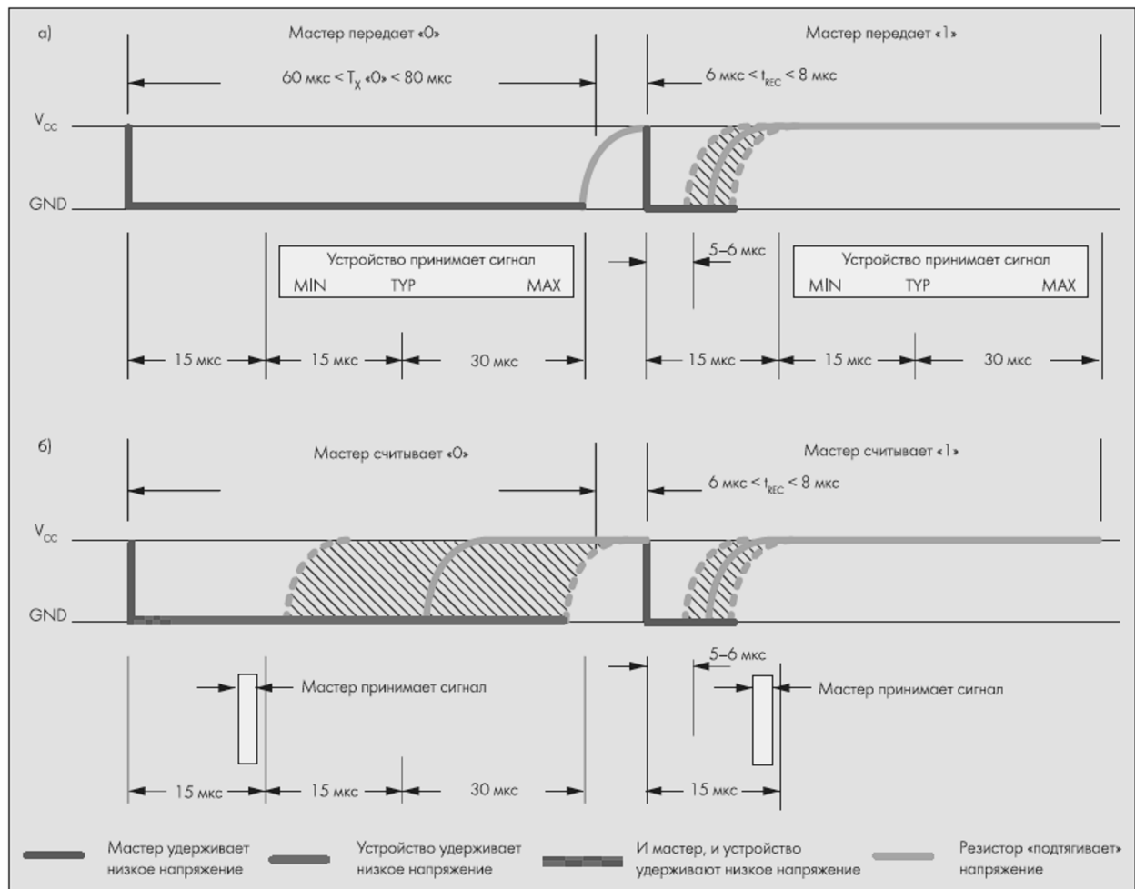
Рис. 4. Передача информационных битов по шине 1-Wire: а – мастер передает сигналы, б – мастер считывает сигналы.
